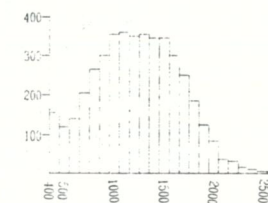
GAUSS-KURVEN
